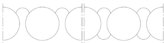
Células circulares com estacas de junção de 35° e um ou dois arcos de conexão.
