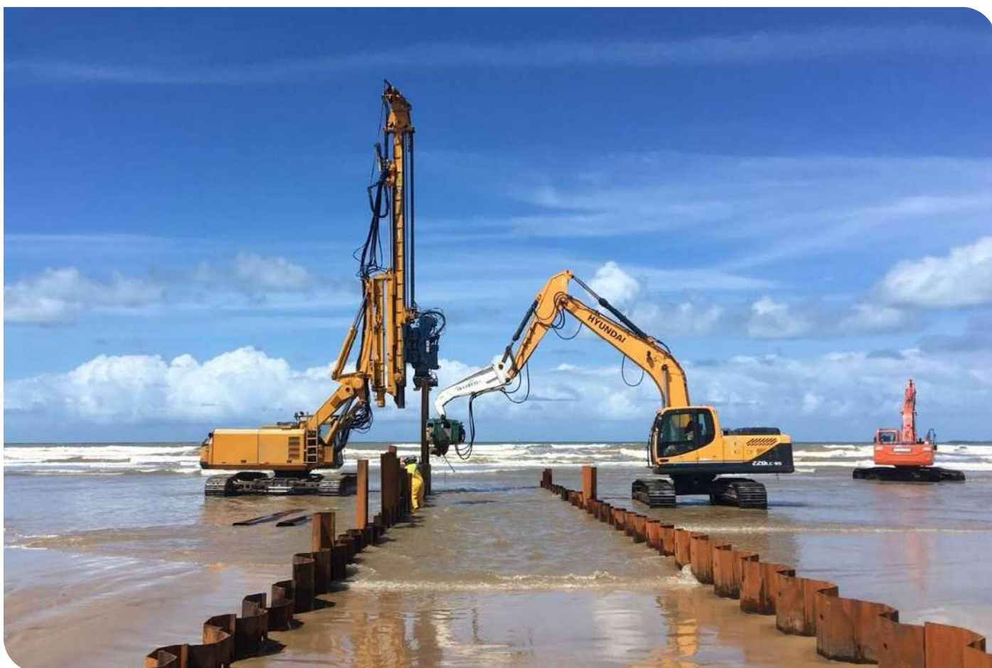
Martelo vibratório acoplado em equipamento com torre guia e em escavadeira Local: UTE Porto de Sergipe
